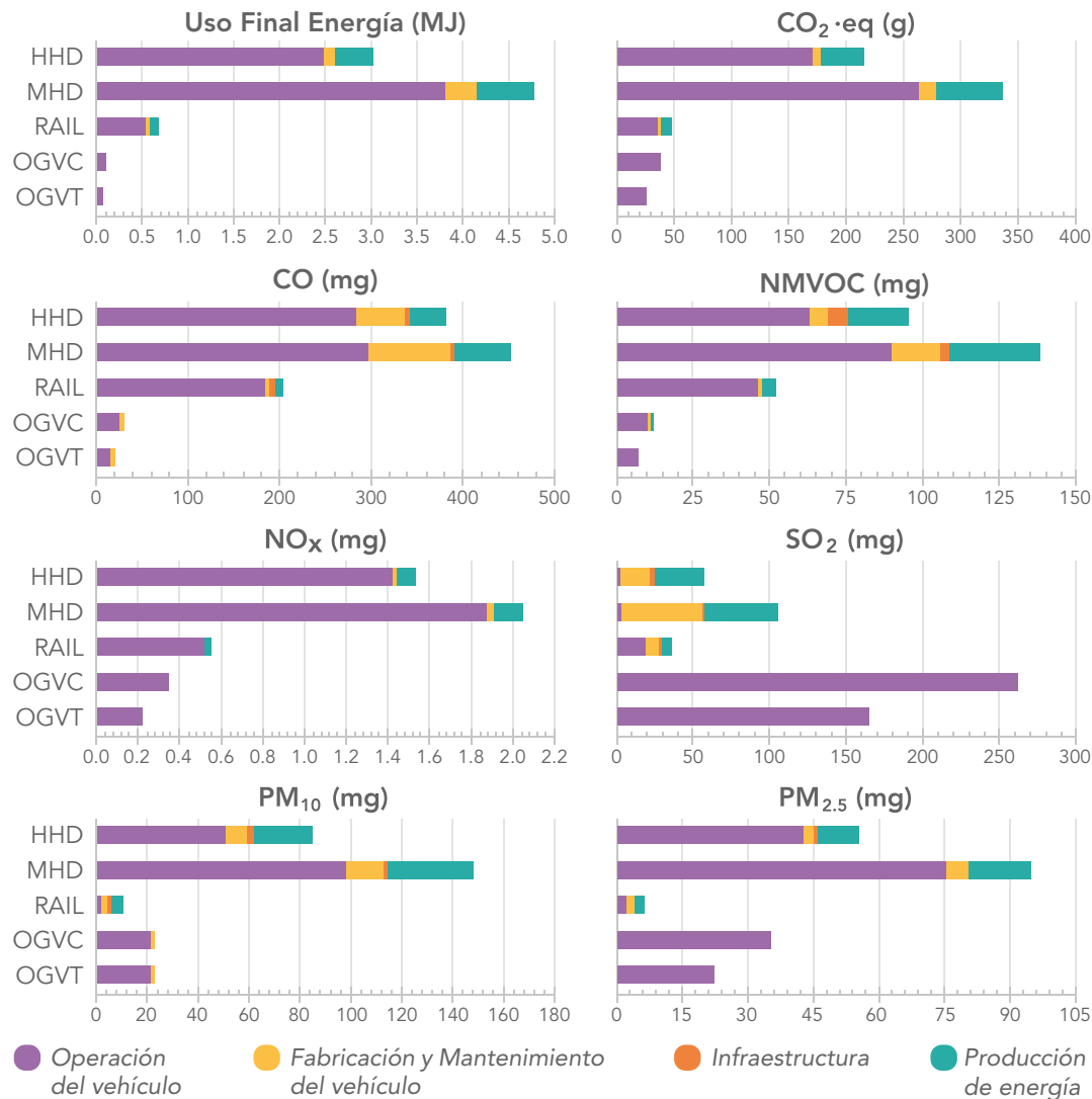
Figura 34. Energía y emisiones usadas en el ciclo de vida por tonelada kilómetro en California.
